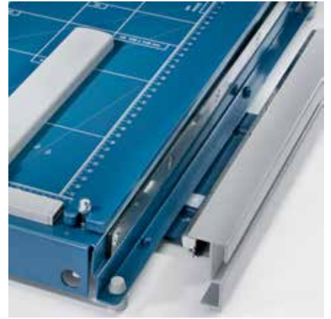
Herausziehbarer Vorderanschlag bis 170 mm mit ausklappbaren Papierhaltern - zum Schneiden von Streifen gleicher Schnittbreite
