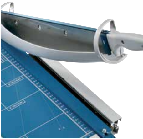
Geschraubtes, geschliffenes Ober- und Untermesser für präzise Schnitte
